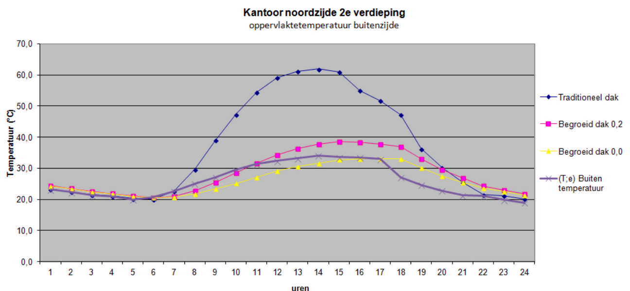
Figuur 5 Simulatie met temperaturen op begroeid dak van kantoorgebouw.
